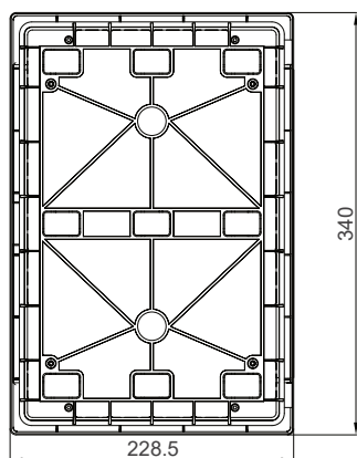
Rozvodnica P-Box pod omiektu, 16 modulová, dvojradová
