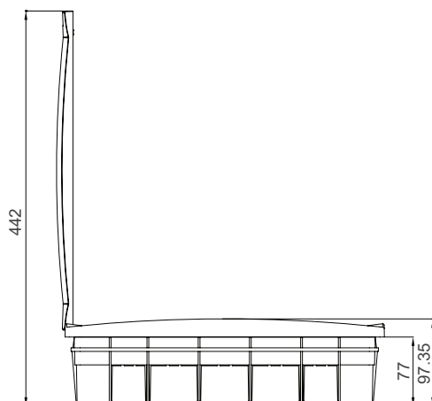
Rozvodnica P-Box pod omiektu, 16 modulová, dvojradová
