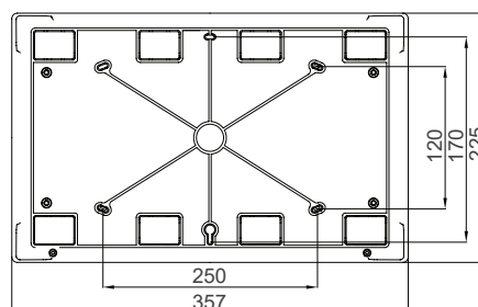
Rozvodnica P-Box nad omiektu, 16 modulová
