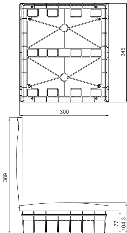
Распределительный щит P-Box под штукатурку, 24 модулей, двойной ряд
