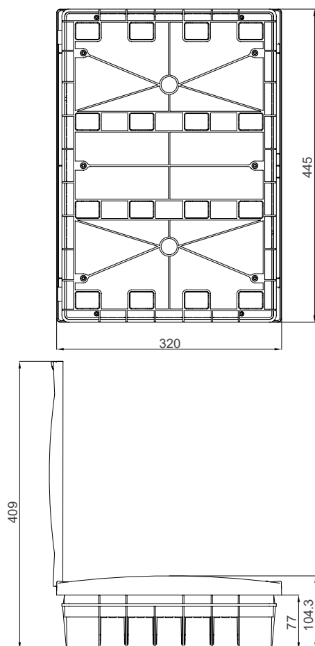
Распределительный щит P-Box под штукатурку, 36 модулей, тройной ряд
