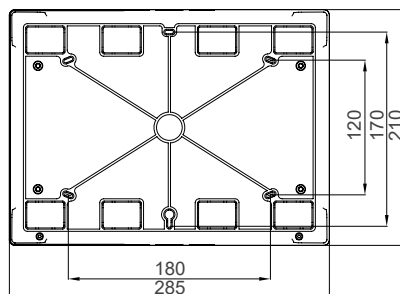
Распределительный щит P-Вох над штукатуркой, 12 модулей
