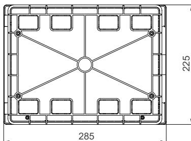
Распределительный щит P-Вох под штукатурку, 12 модулей
