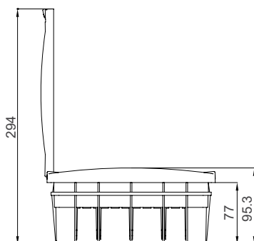
Распределительный щит P-Вох под штукатурку, 12 модулей
