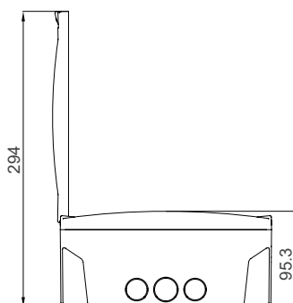
Распределительный щит P-Вох над штукатуркой, 12 модулей
