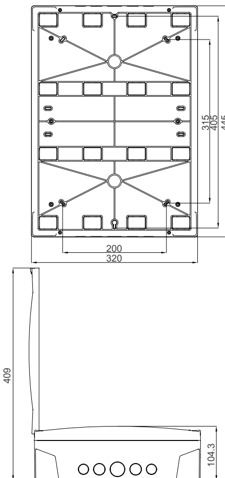
Распределительный щит P-Box над штукатуркой, 36 модулей, тройной ряд
