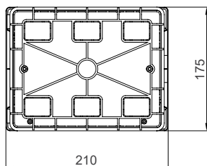
Распределительный щит P-Вох под штукатурку, 8 модулей
