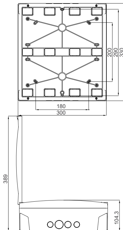
Распределительный щит P-Box над штукатуркой, 24 модулей, двойной ряд
